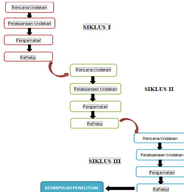
Gambar 1. Siklus Penelitian
